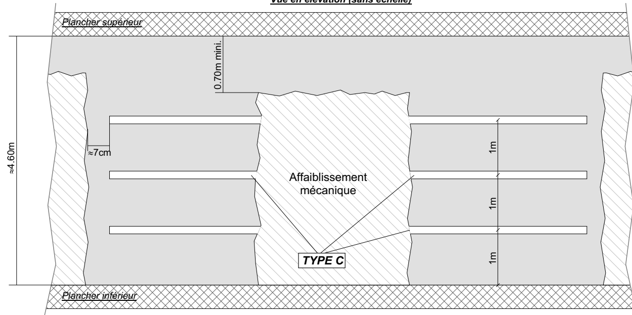
Vue en élévation (sans échelle)
